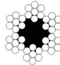
6×7+FC
