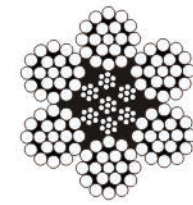
6×19+IWRC
