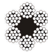
6×19+FC
