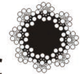
8×19 ( S ) +FC
