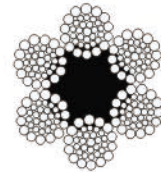
6×36 ( WS ) +FC
