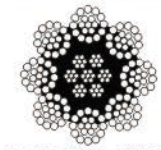
8×19 ( W ) +IWRC
