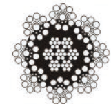
8×19 ( S ) +IWRC
