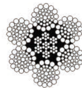
6×36 ( WS ) +IWRC
