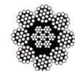
8×19 ( W ) +IWRC
