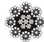
8×19 ( S ) +IWRC
