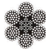
6×37+IWRC
