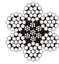
6×19+IWRC
